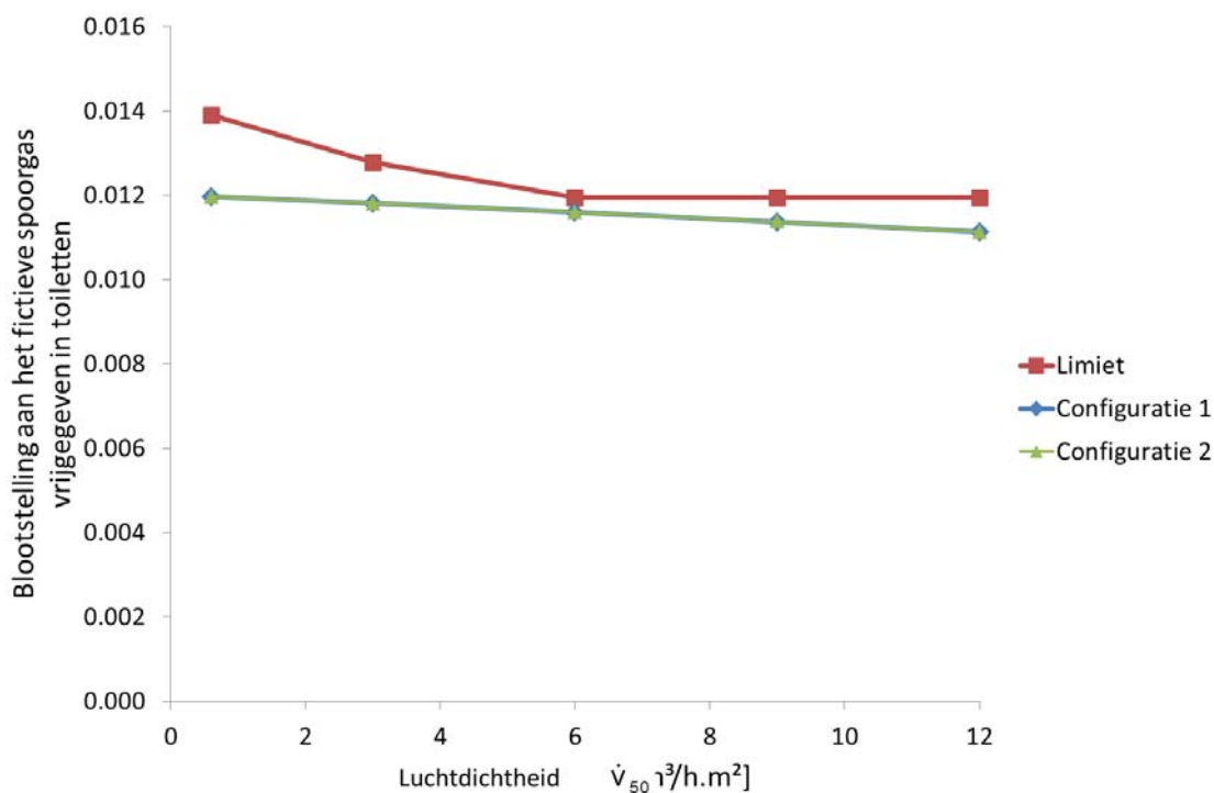
Figuur 3: de globale blootstelling aan een fictief spoorgas vrijgegeven in toiletten op ogenblikken van bezetting voor de twee configuraties van het vraaggestuurde ventilatiesysteem Duco Comfort Plus System
