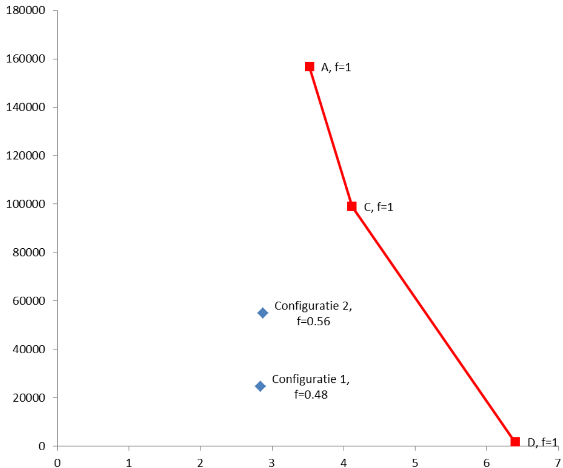
Figuur 4: Warmteverliezen door bewuste ventilatie gedurende de verwarmingsperiode en binnenluchtkwaliteit (CO 2 )
