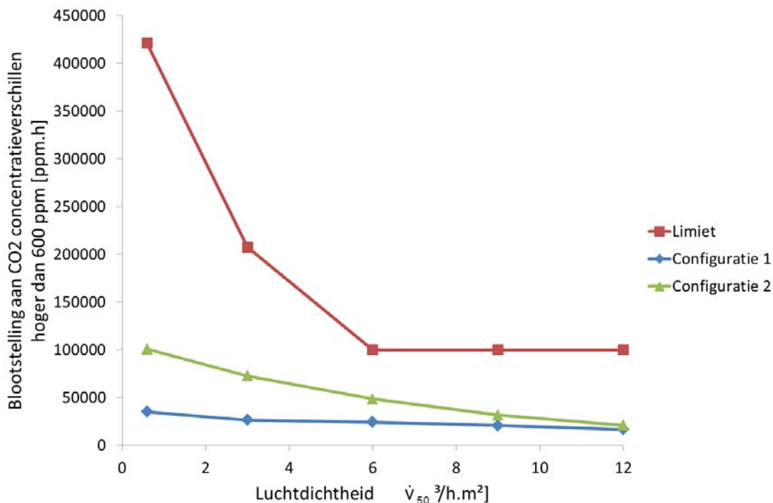
Figuur 2: de globale blootstelling aan CO 2 concentratieverschillen hoger dan 600 ppm voor de twee configuraties van het vraaggestuurde ventilatiesysteem Duco Comfort Plus System
