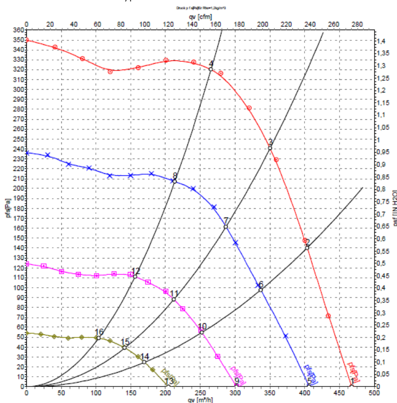
Figuur 1: ventilatorcurve
