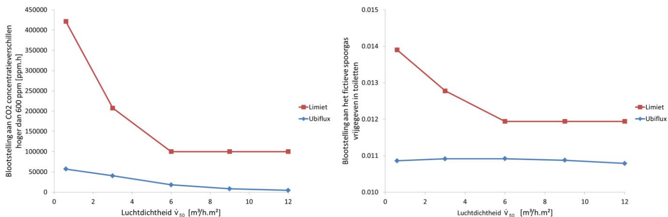
Figuur 1: Blootstellingen aan CO 2 (links) en aan het fictieve spoorgas vrijgegeven in toiletten (rechts)
