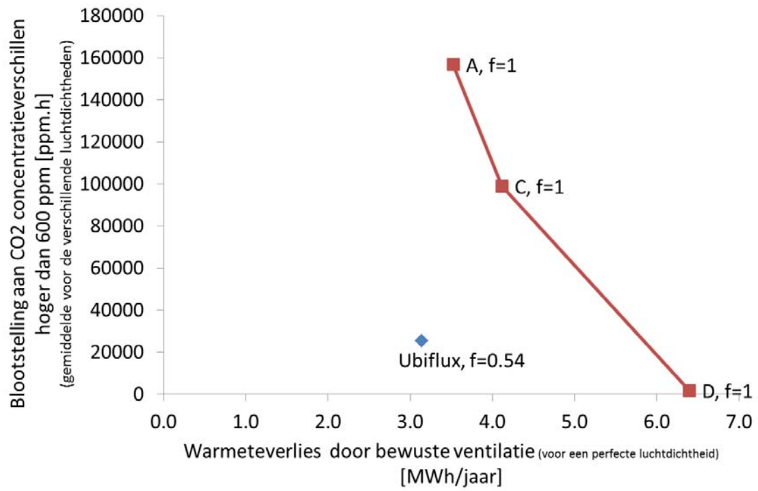
Figuur 2: Prestaties voor warmteverlies en binnenluchtkwaliteit
